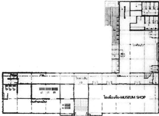
แบบแปลน อาคารปูน ชั้น ๑
